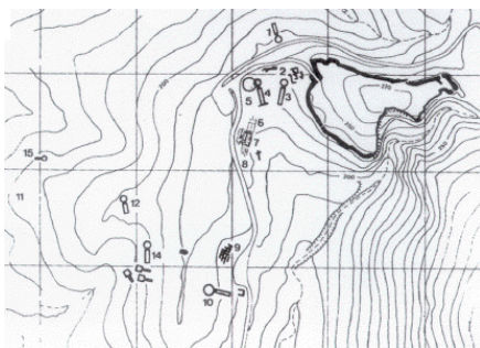
plattegrond Mykenai
